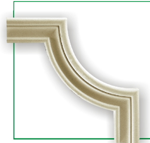
CF 3063-B 180x180x15mm 7 1/16 x 7 1/16 x 5/16"
